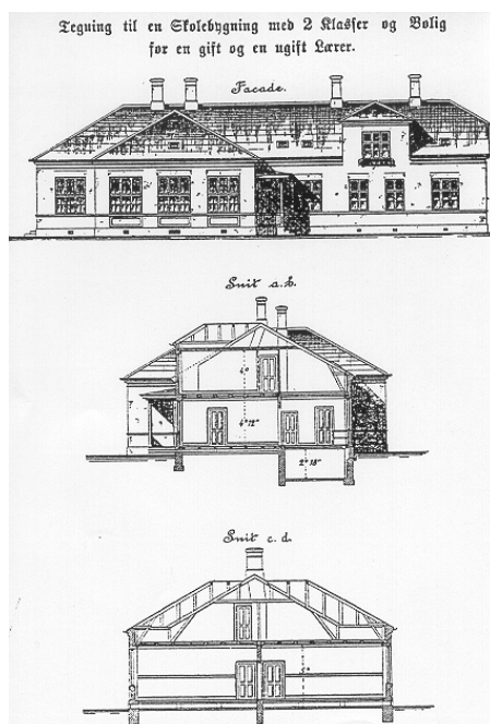
Christian Thurens statslige mønstertegninger, 1900
