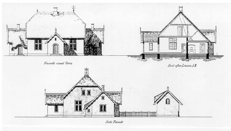
J.D. Herholdts statslige mønstertegninger, 1857
