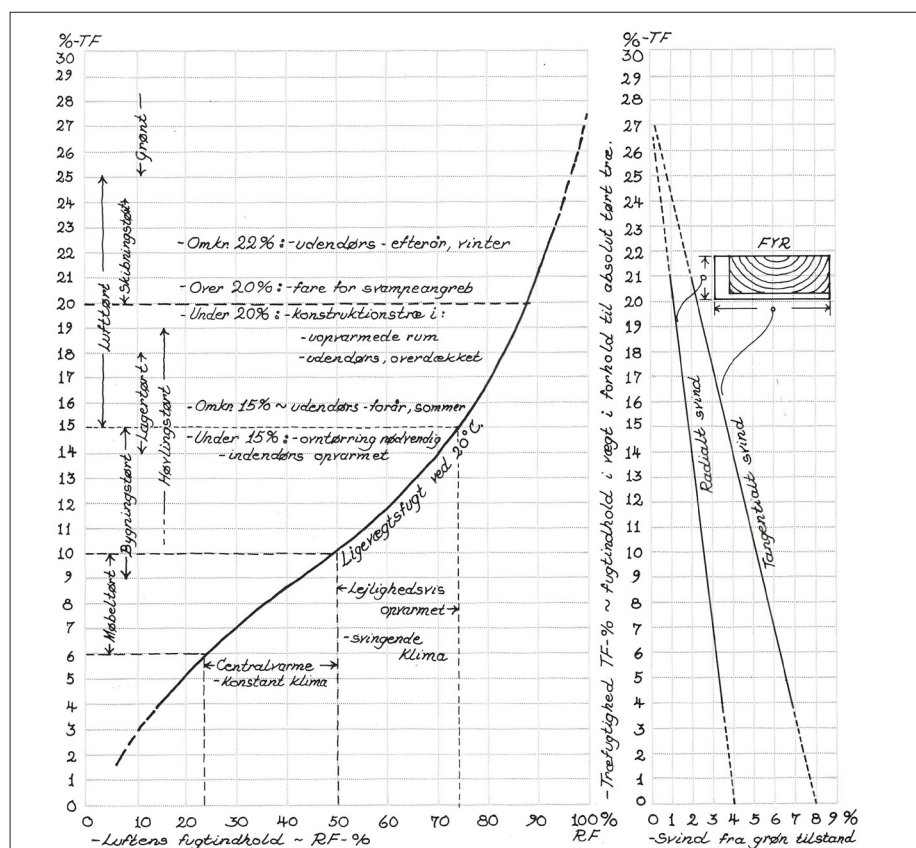
Kurver for fugtindhold og ligevægtsfugt samt for svind. Efter Th. Thomassen: Træ og træmaterialer.ring
