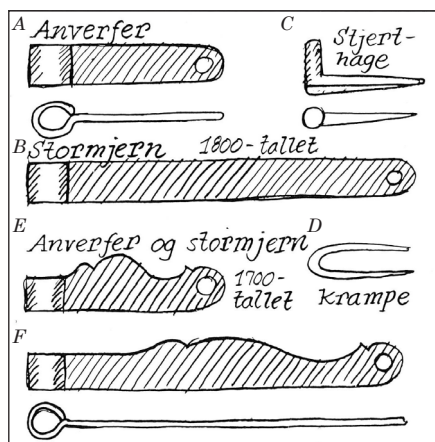
Hullet slås i det glødende jern med et lokkestempel. Huller i jern udført på denne måde er mere modstandsdygtige overfor rustangreb end almindelige borede huller. Det skyldes, at jernet får en mere kompakt struktur og en beskyttende glødeskal.
