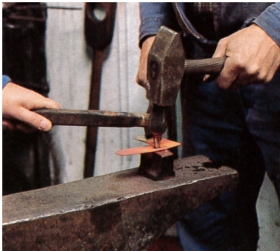
Hullet slås i det glødende jern med et lokkestempel. Huller i jern udført på denne måde er mere modstandsdygtige overfor rustangreb end almindelige borede huller. Det skyldes, at jernet får en mere kompakt struktur og en beskyttende glødeskal.
