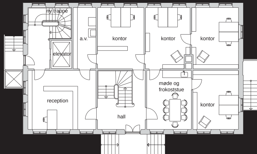
Stueetage - Fremtidige forhold
