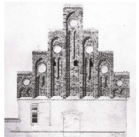
Gotisk kamtakket gavl med høje spidsbueblændinger. Stengade 66 i Helsingør, formentlig opført 1517. Opmåling i Eldre nordisk Arkitektur .
