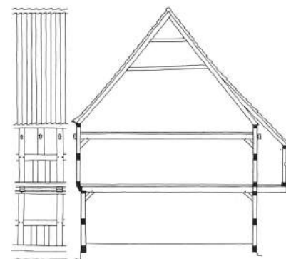
Svalegangshus fra 1723. Tværsnit og facadefag. Minimalt stokværksfremspring. Øverste bjælker tappet i stolper under rem. Lodrette dokker i tavl. Tegning af LP.
