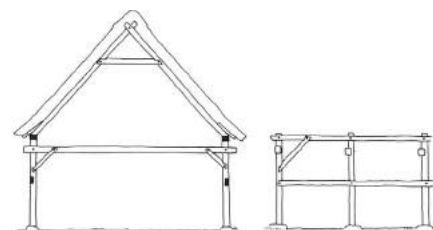
Svalegangshus fra 1723. Tværsnit og facadefag. Minimalt stokværksfremspring. Øverste bjælker tappet i stolper under rem. Lodrette dokker i tavl. Tegning af LP.
