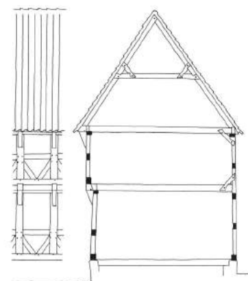
Renæssancehus fra 1583. Tværsnit og facadefag. Lille knægtbåret stokværksfremspring mod gade og højstolper i gårdside. Øverste bjælker over rem. Tegning af LP.
