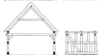
Tværsnit og langside i landbygninger. Øverst nordøstdansk (sidebånd og glammede bjælker), nederst vestdansk (svært bindingsværk på fodrem). Tegning af LP.
