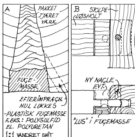
Tjærekit fremstilles af træetjære, iblandet slemmet kridt til en kitagtig konsistens.
