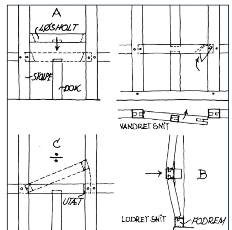
Skarring af stolpefod i konstruktion uden fodrem. Med små kiler spændes samlingen tæt og til bæring. Der understøttes. Efter betonens afhærdning fjernes kilerne, og hullet udstøbes.
