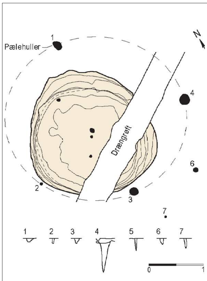
Fig. 6. HØM106 oversigtsplan hytte 2: Plantegning af hyttegrube og tilknyttede stagehuller (hytte 2 fra Nivå og Lollikhuse). Tegning: O.L. Jensen, Hørsholm Egns Museum
